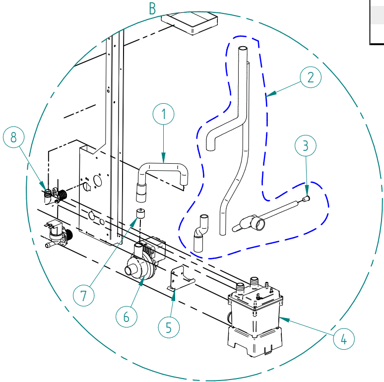
DETALLE B
