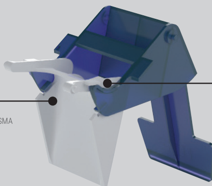
ROCKING DISPENSING MECHANISM EMPUJADOR APERTURA COMPUERTA
