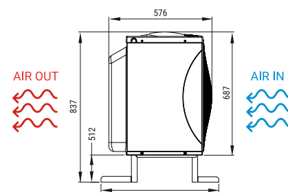
RIGHT SIDE VIEW VISTA LATERAL DERECHA
