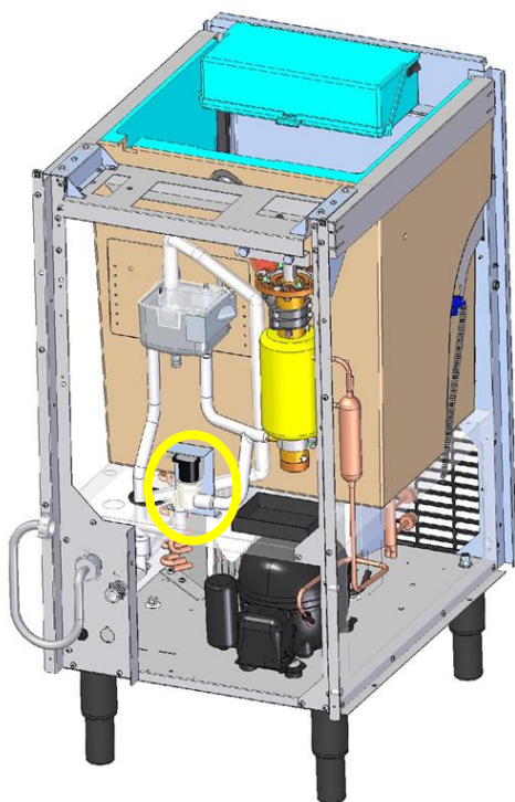
Machine compacte
