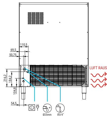
RÜCKANSICHT
