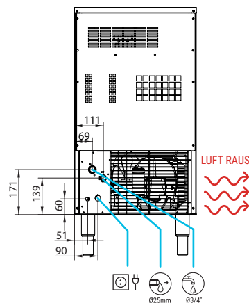
RÜCKANSICHT
