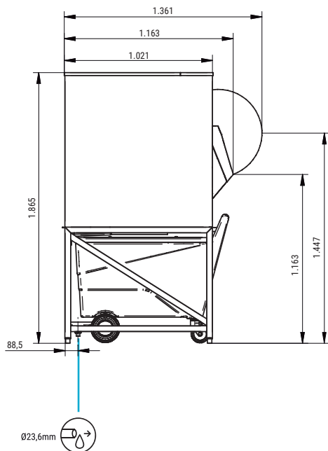
RIGHT SIDE VIEW VISTA LATERAL DERECHA
