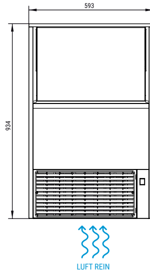
FRONTANSICHT
