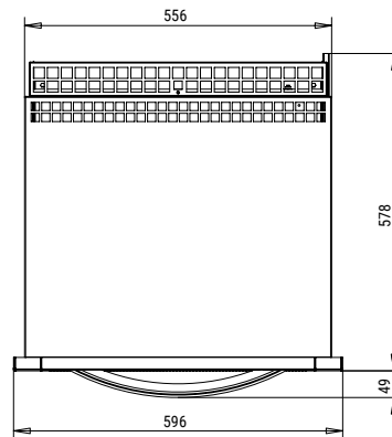
UNTERE ANSICHT
