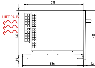
UNTERE ANSICHT
