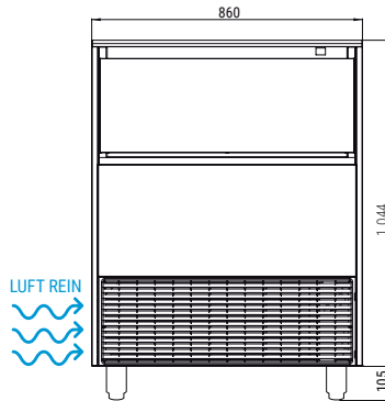
FRONTANSICHT
