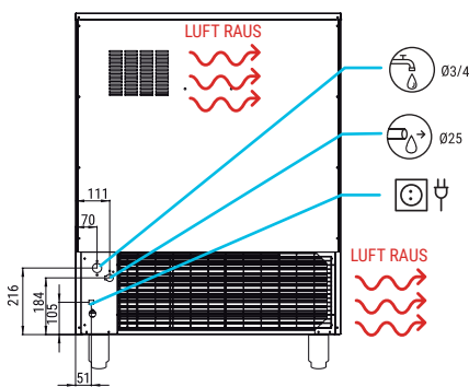
RÜCKANSICHT
