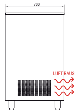
LINKE SEITENSICHT
