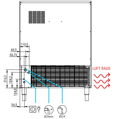
RÜCKANSICHT
