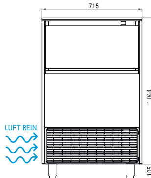
FRONTANSICHT
