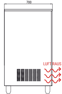
LINKE SEITENANSICHT
