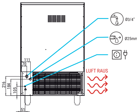
RÜCKANSICHT
