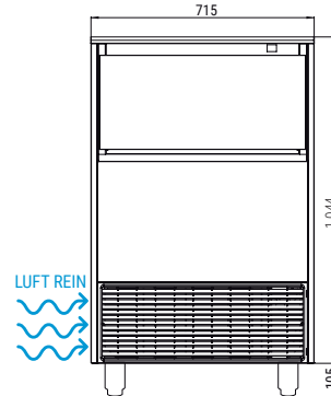
FRONTANSICHT
