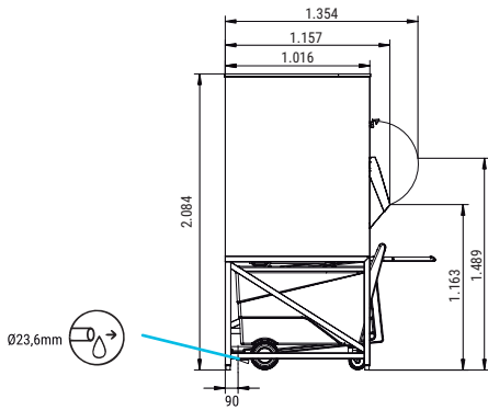
RIGHT SIDE VIEW VISTA LATERALE SINISTRA
