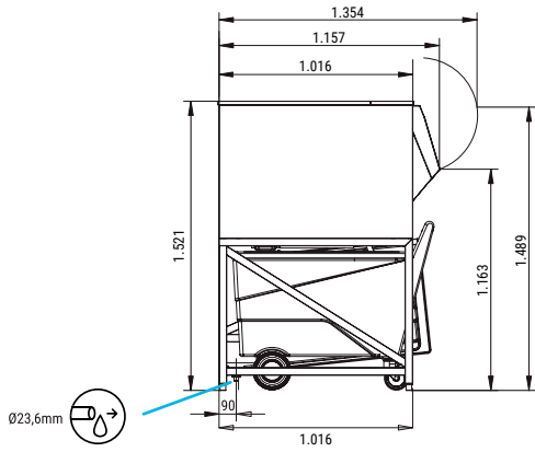
RIGHT SIDE VIEW VISTA LATERALE SINISTRA
