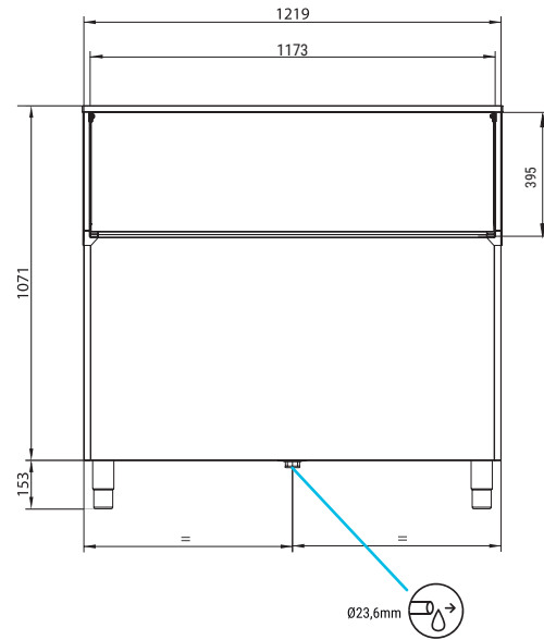
FRONTANSICHT
