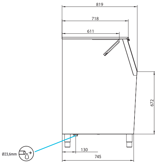
RECHTE SEITENANSICHT
