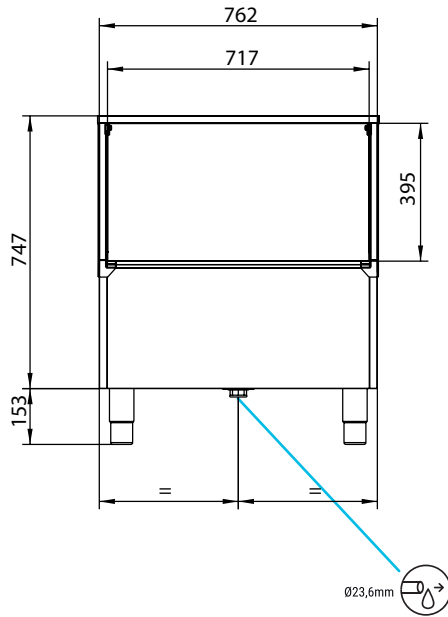
FRONTAL VIEW VUE DE FACE
