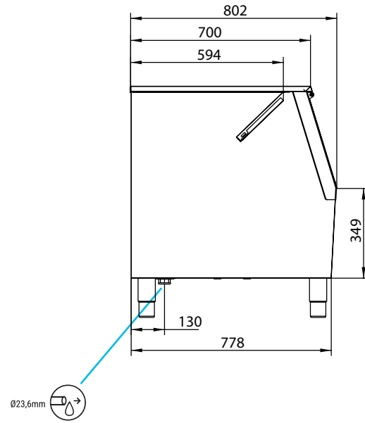
LEFT SIDE VIEW VUE LATÉRALE IZQUIERDA
