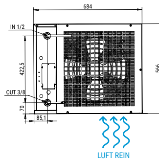
RECHTE SEITENSANSICHT
