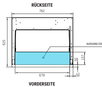
ZENTRALE QUERSCHNITTSANSICHT DER BASIS
