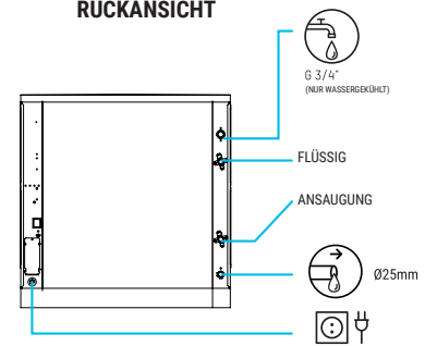
RÜCKANSICHT
