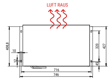
UNTERE ANSICHT
