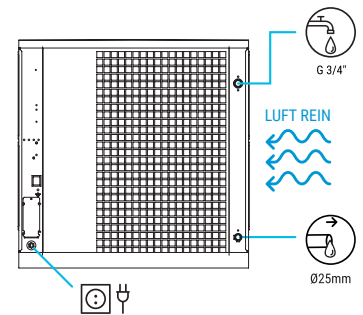
RÜCKANSICHT
