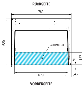
ZENTRALE QUERSCHNITTSANSICHT DER BASIS
