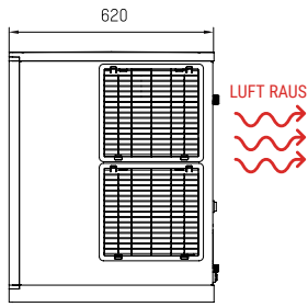
RECHTE SEITENANSICHT
