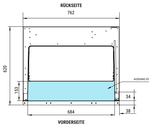
ZENTRALE QUERSCHNITTSANSICHT DER BASIS
