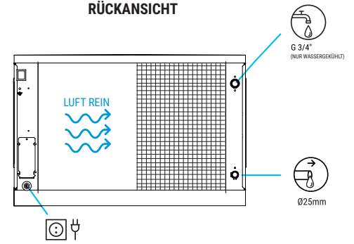
RÜCKANSICHT
