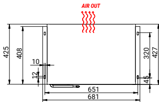
TOP VIEW VISTA EN PLANTA
