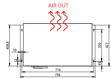
TOP VIEW VUE EN PLAN
