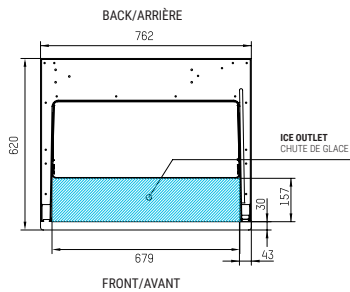
CENTRAL CROSS SECTION VIEW OF THE BASE VUE DE LA BASE DEPUIS LA SECTION CENTRALE
