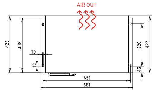
TOP VIEW VUE EN PLAN
