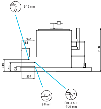
RECHTE SEITENANSICHT
