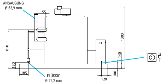
QUERSCHNITT-ANSICHT DER BASIS
