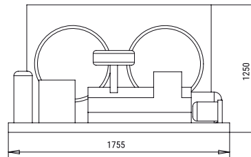
RIGHT SIDE VIEW VISTA LATERALE DESTRA
