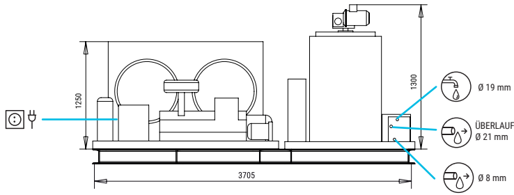
FRONTANSICHT
