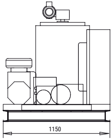
RECHTE SEITENANSICHT
