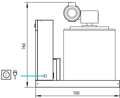
RECHTE SEITENSICHT
