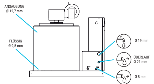
LINKE SEITENSICHT
