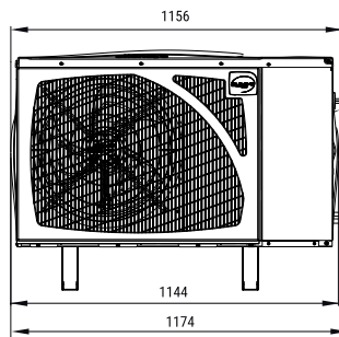
RECHTE SEITENSICHT
