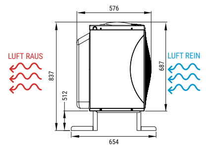
RECHTE SEITENSICHT
