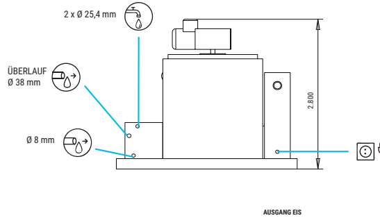
QUERSCHNITT-ANSICHT DER BASIS
