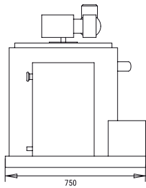
RECHTE SEITENANSICHT
