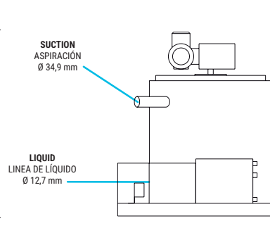
LEFT SIDE VIEW VISTA LATERAL IZQUIERDA
