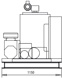
RECHTE SEITENANSICHT
