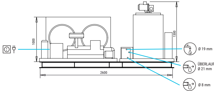
QUERSCHNITT-ANSICHT DER BASIS
