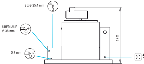
FRONTANSICHT
