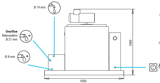
FRONTAL VIEW VUE DE FACE
