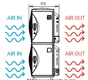
RIGHT SIDE VIEW VUE LATÉRALE DROITE
