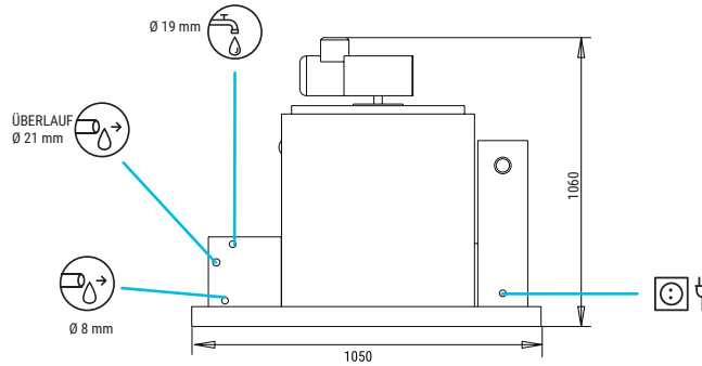
FRONTANSICHT
