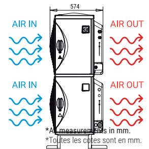
RIGHT SIDE VIEW VUE LATÉRALE DROITE
