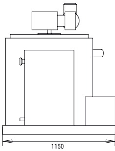
QUERSCHNITT-ANSICHT DER BASIS
