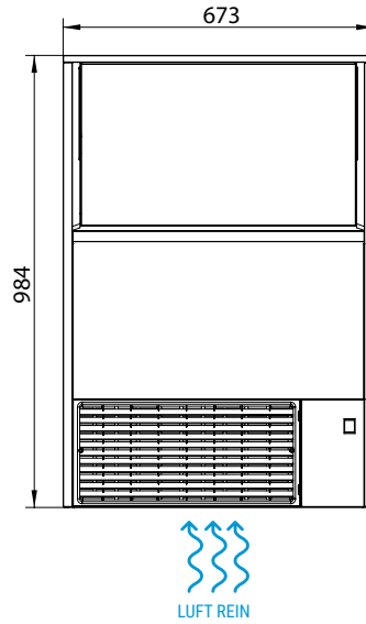
FRONTANSICHT
