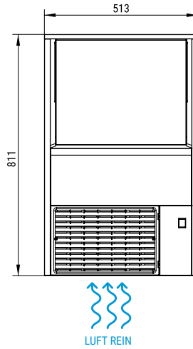
FRONTANSICHT
