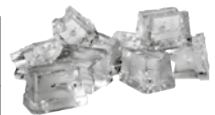
ALFA 14/19gr 36 mm (W) x 26 mm (D) x 23 mm (H) Average dimensions Dimensiones promedio
