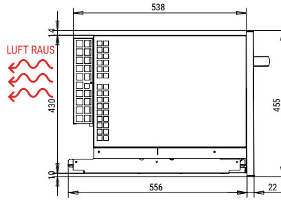
UNTERE ANSICHT
