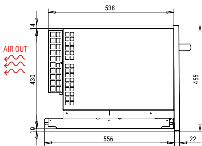
RIGHT SIDE VIEW VUE LATÉRALE DROITE
