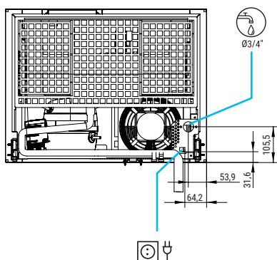
REAR VIEW VUE ARRIÈRE
