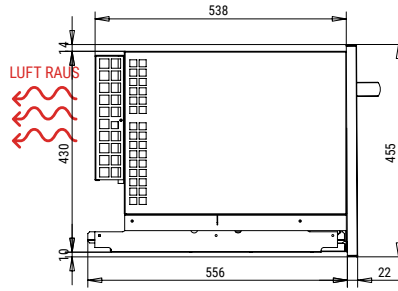
UNTERE ANSICHT
