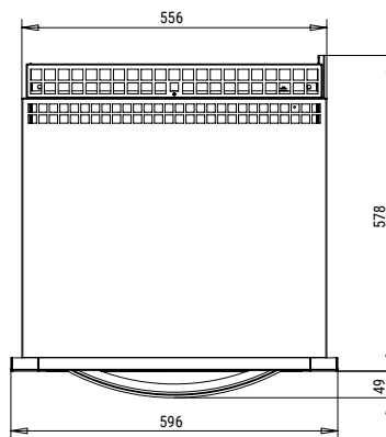
UNTERE ANSICHT
