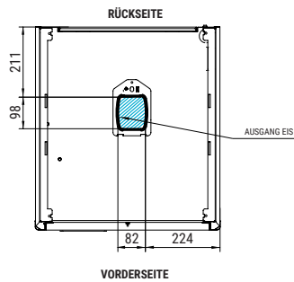
ZENTRALE QUERSCHNITTSANSICHT DER BASIS
