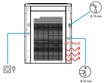
RÜCKANSICHT
