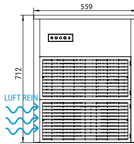
FRONTANSICHT
