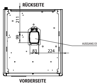
ZENTRALE QUERSCHNITTSANSICHT DER BASIS
