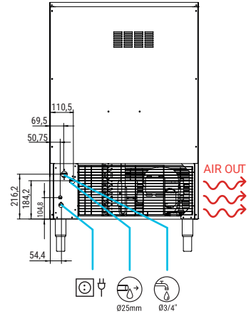
RÜCKANSICHT
