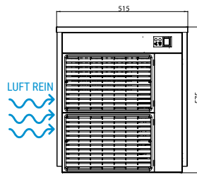
FRONTANSICHT
