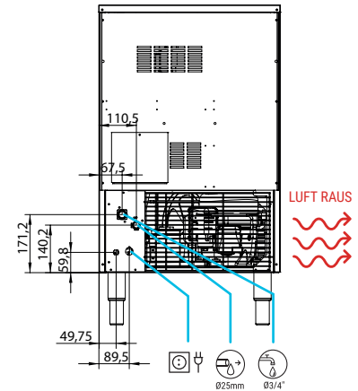
RÜCKANSICHT
