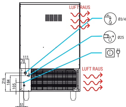
RÜCKANSICHT
