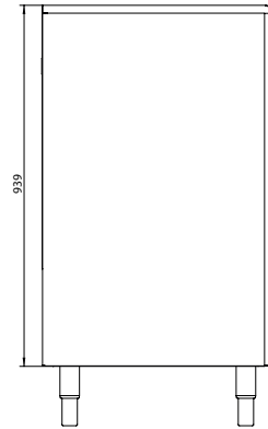
LEFT SIDE VIEW VUE LATÉRALE GAUCHE
