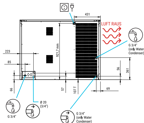
RÜCKANSICHT
